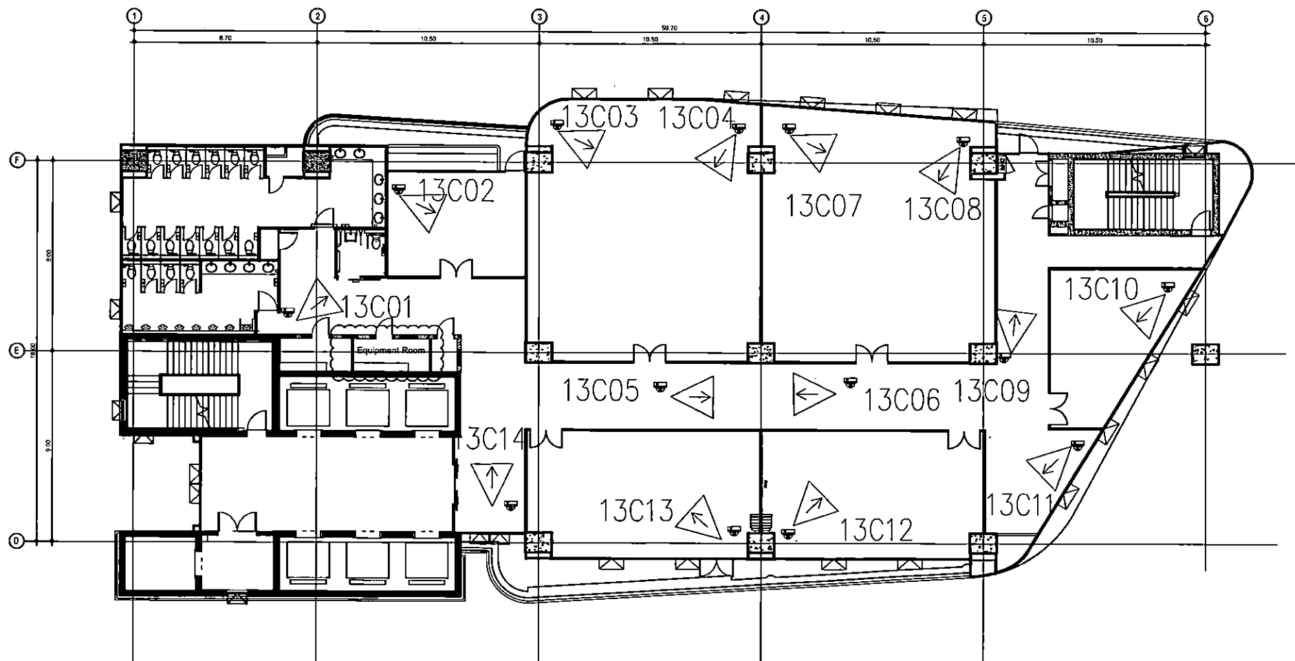
แบบแสดงตำแหน่งติดตั้งกล่องวงจรปิด
