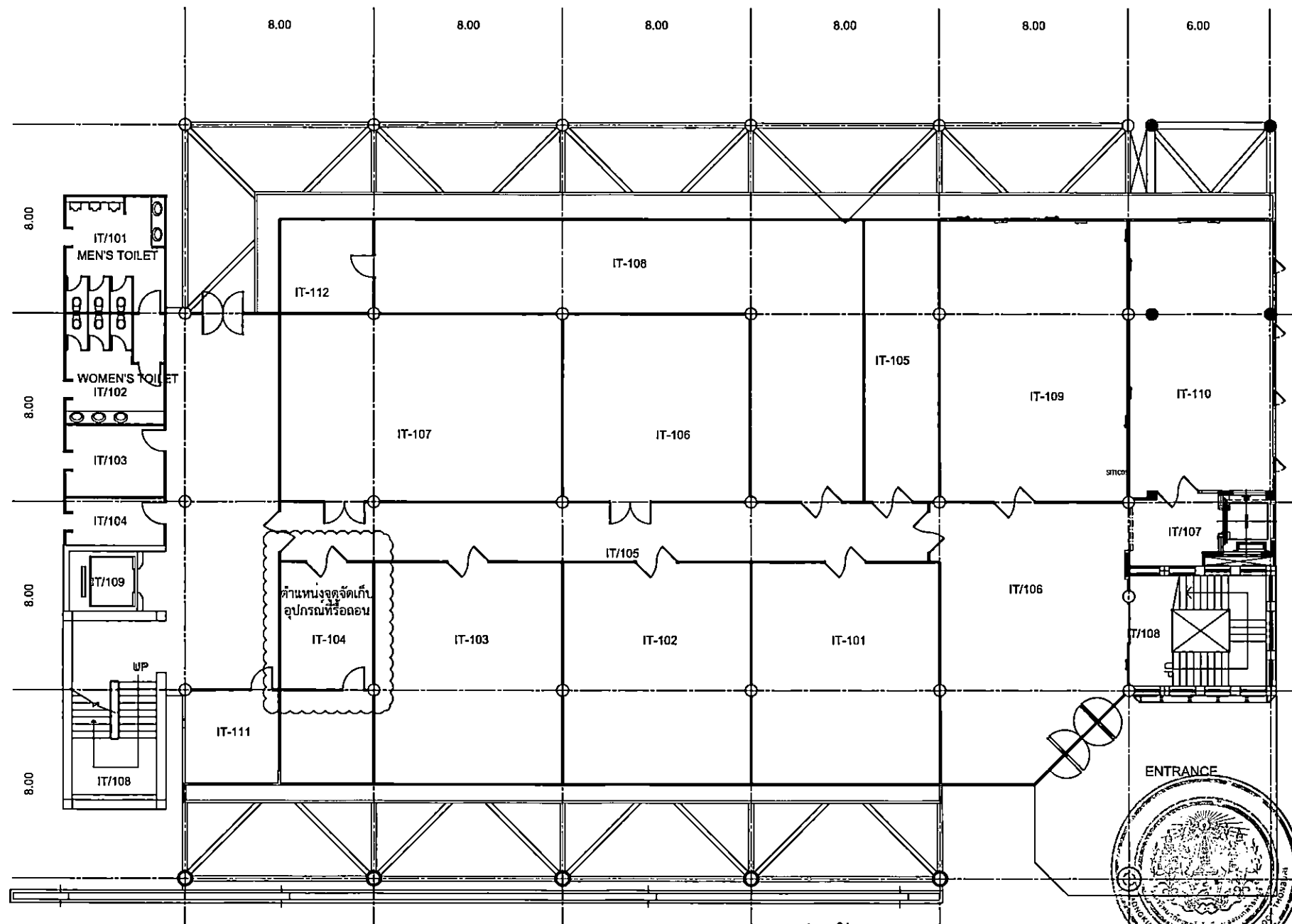
แบบแสดงตำแหน่งจุดจัดเก็บอุปกรณ์ที่รื้อถอน
