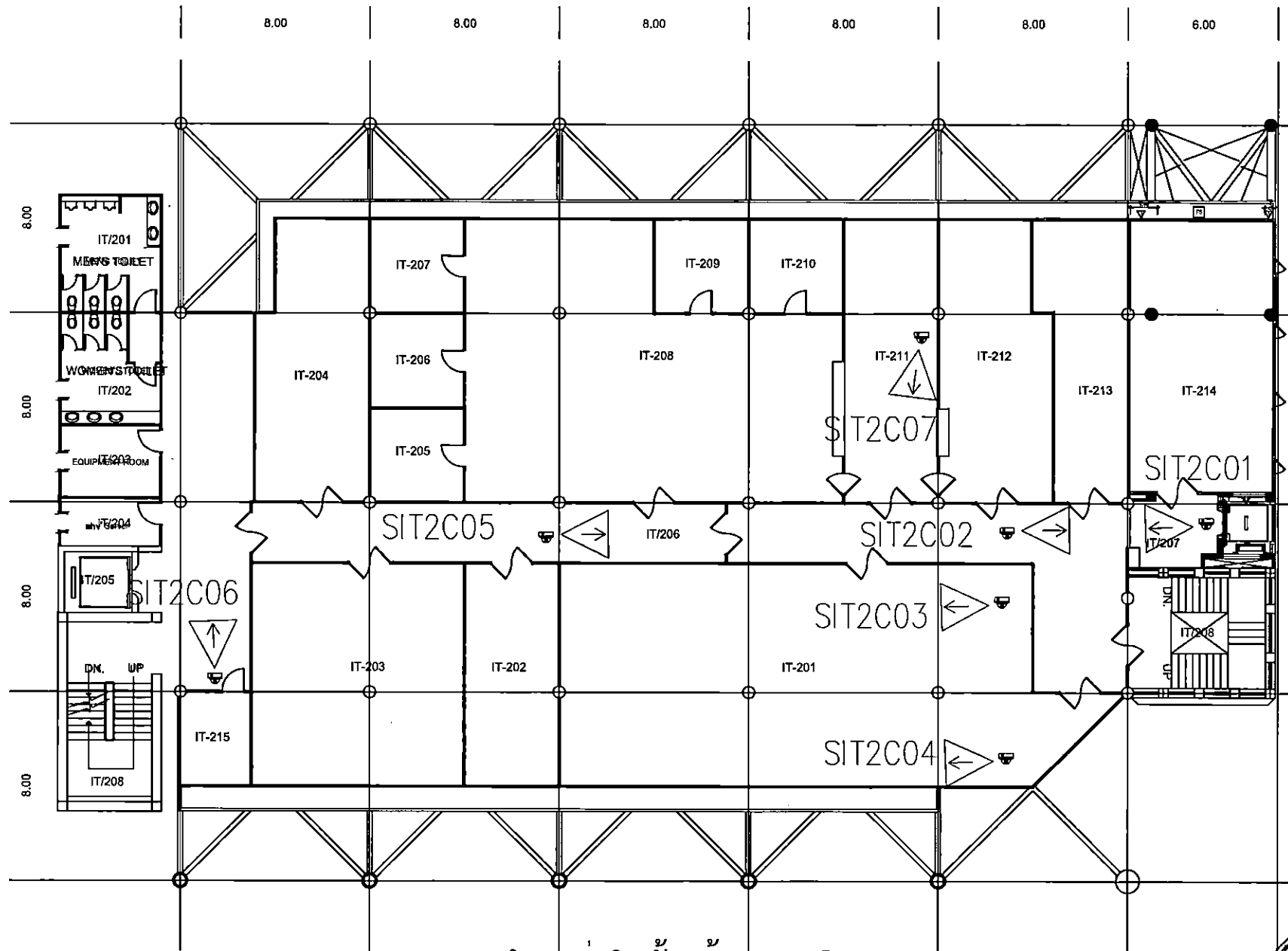
แบบแสดงตำแหน่งติดตั้งกล่องวงจรปิด
