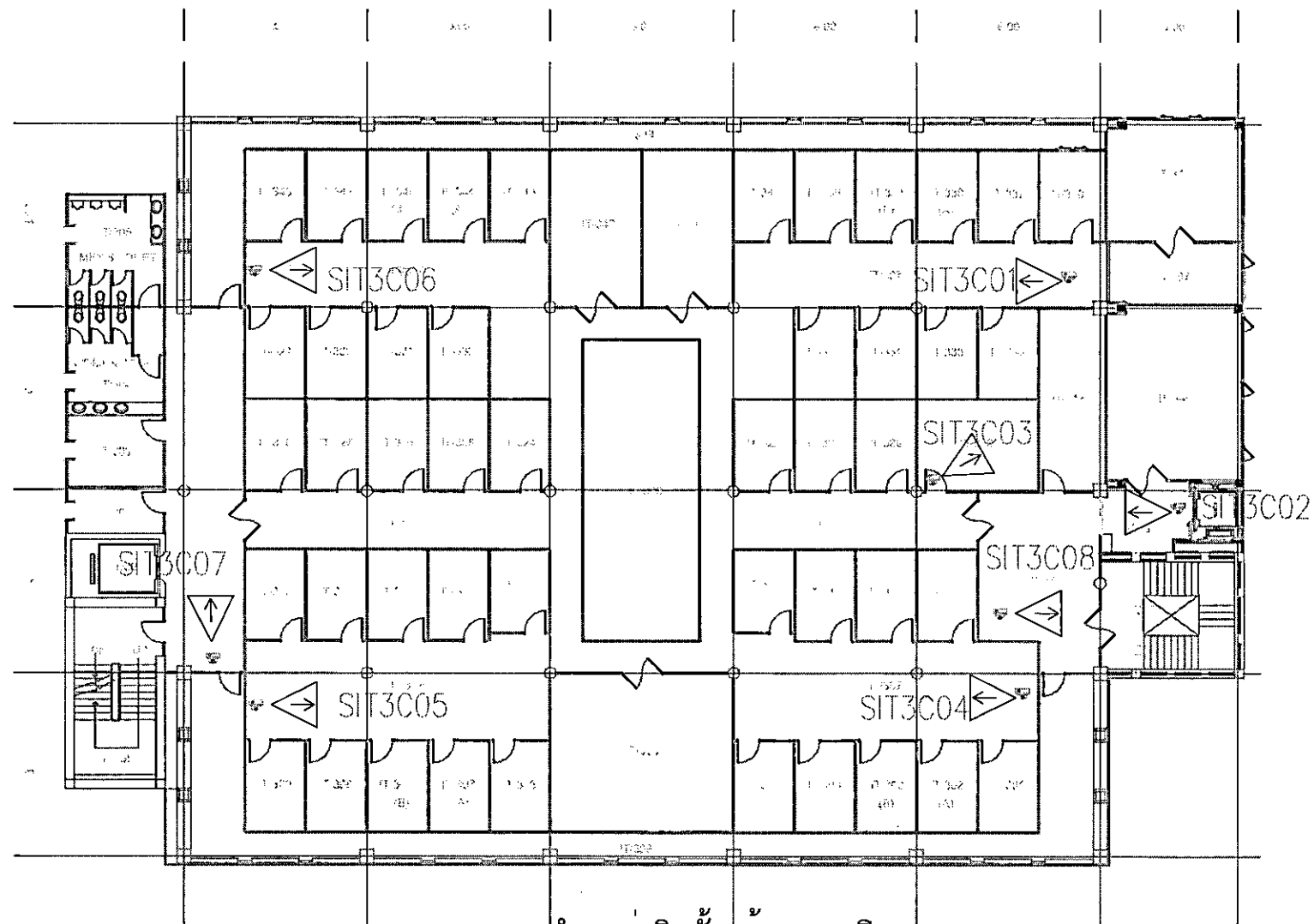
แบบแสดงตำแหน่งติดตั้งกล้องวงจรปิด
