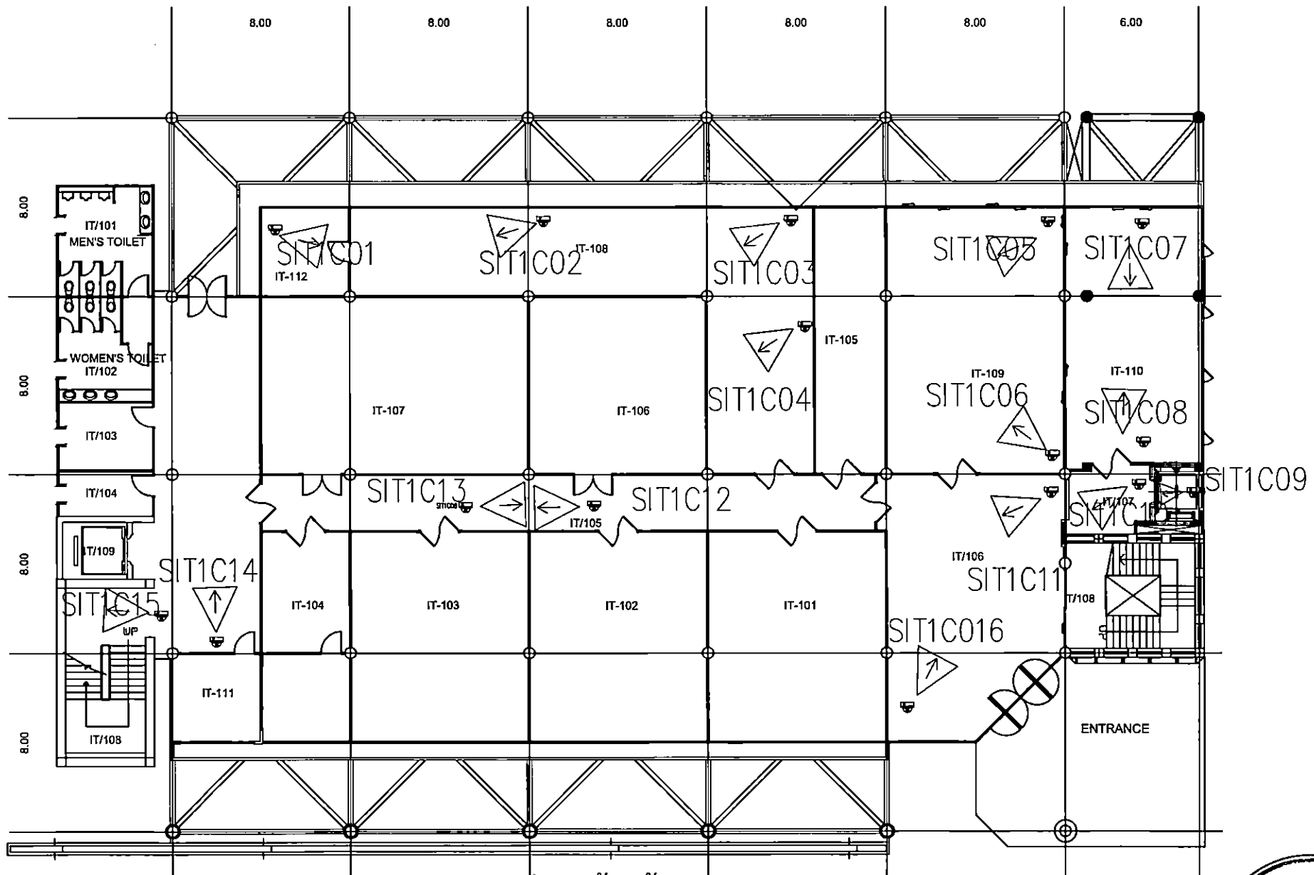
แบบแสดงตำแหน่งติดตั้งกล่องวงจรปิด
