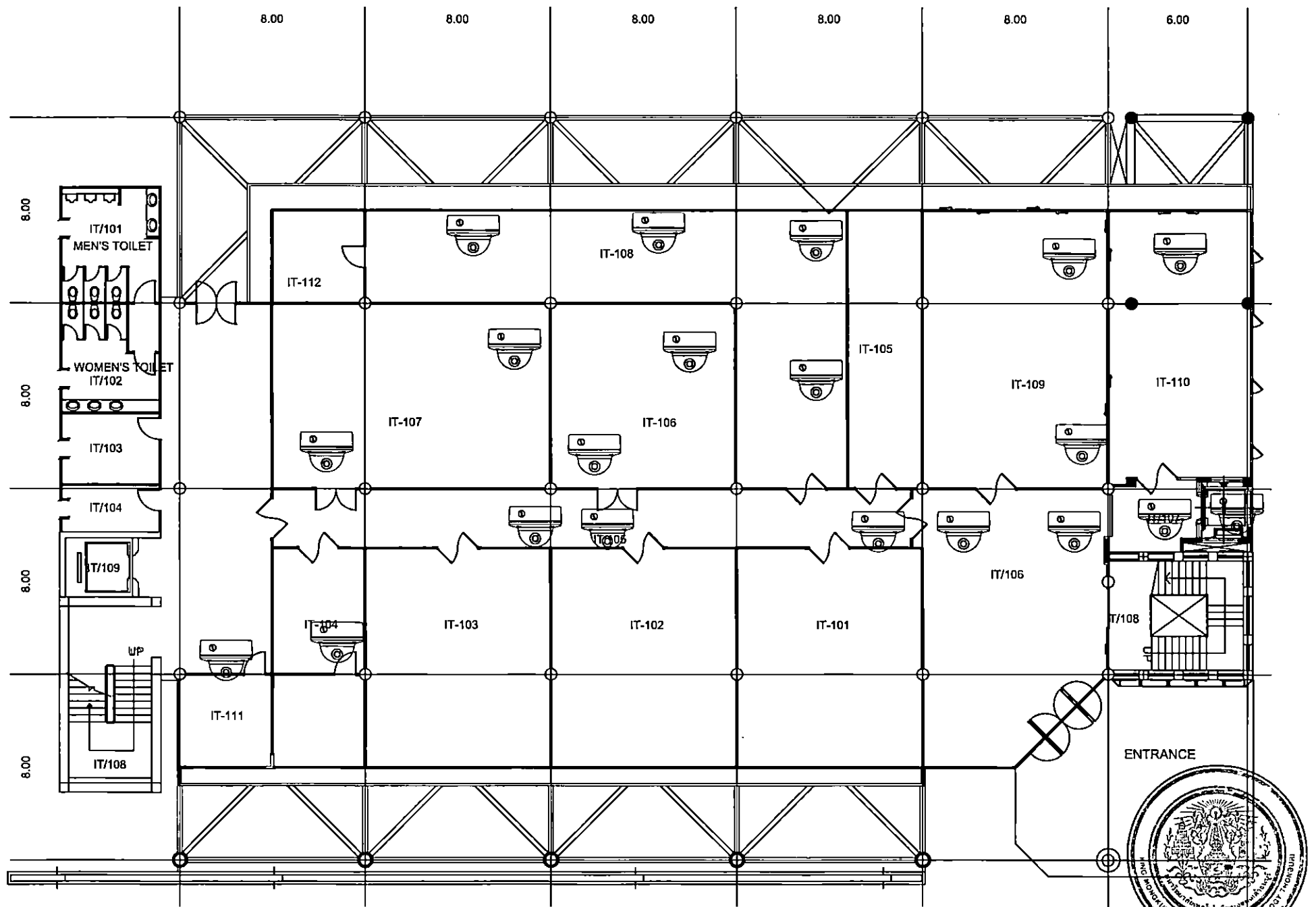
แบบแสดงตำแหน่งรื้อถอนกล่องวงจรปิดเดิม ชั้น 1 อาคารคณะเทคโนโลยีสารสนเทศ มหาวิทยาลัยเทคโนโลยีพระจอมเกล้าธนบุรี
